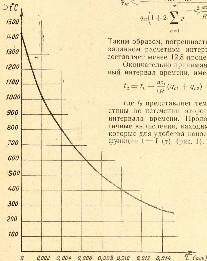
Рис. 1. Изменение температуры частицы на металлизированной поверхности.
