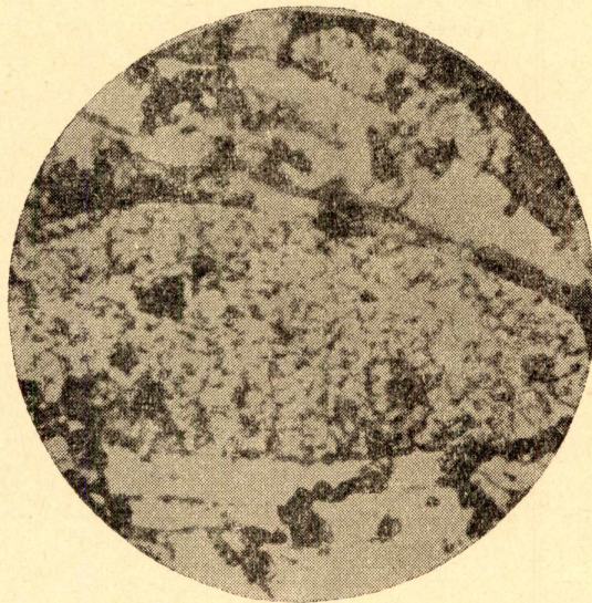
Рис. 2. Структура капли — мелкоигольчатый мартенсит. (сталь У12А.) \times 400 .
