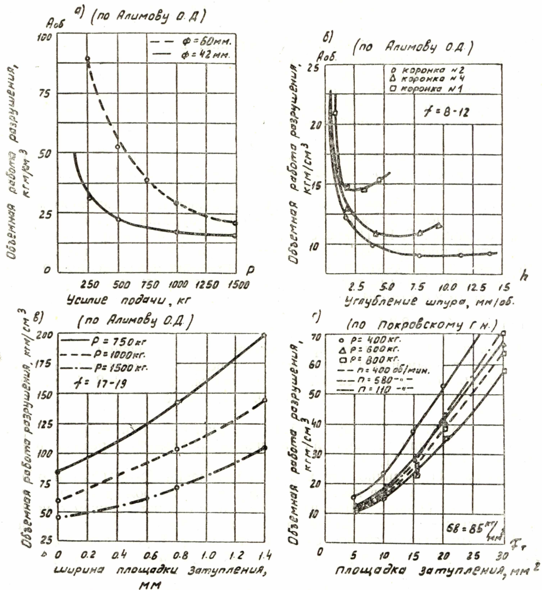
Рис. 11. Зависимость объемной работы разрушения от усилия подачи (а), углубления шпура за оборот (б) и от степени износа резьбы (в) и (г).
