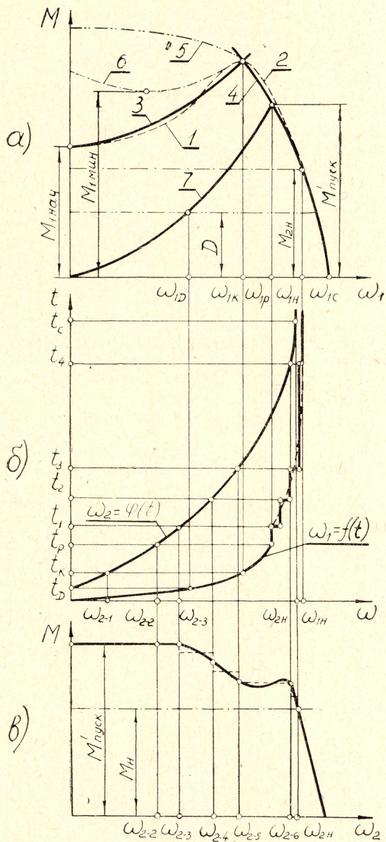
Рис. 2. Механическая характеристика асинхронного электродвигателя (а); характер изменения скоростей ведущего и ведомого валов турбомуфты в процессе разгона (б) и ее обобщенная механическая характеристика (в).
