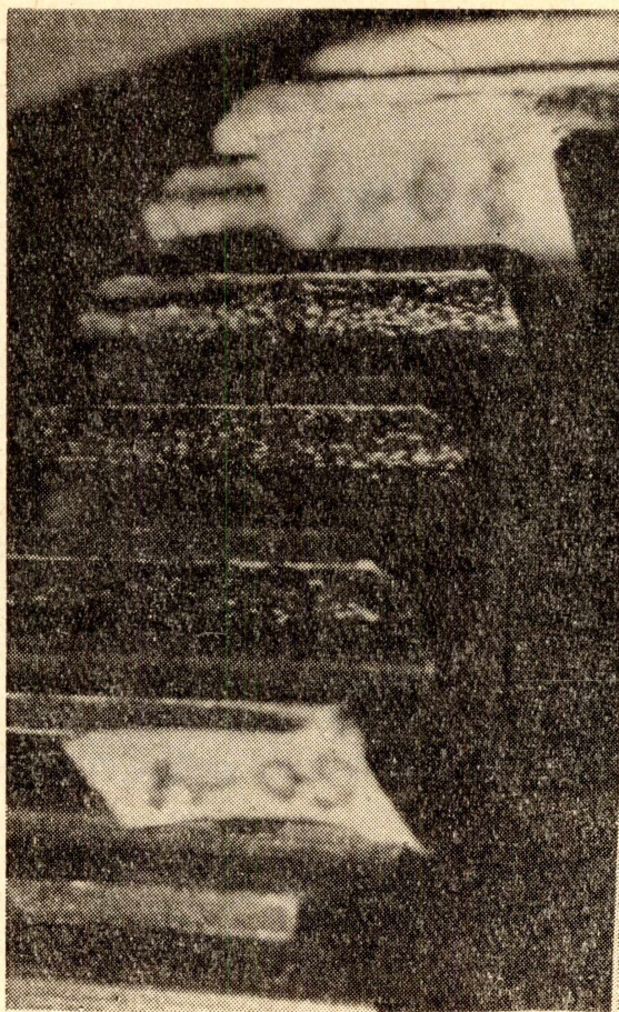
Рис. 3. Колесо первой группы, ведущее. Нагрузка резко переменная от \sigma_k = 48 \text{ кг/мм}^2 до \sigma_k = 80 \text{ кг/мм}^2 .
