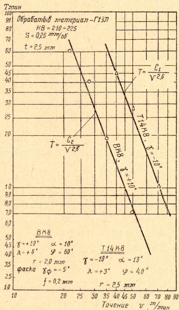
Рис. 2. Зависимости "Т—V" при точении стали Г13Л.
