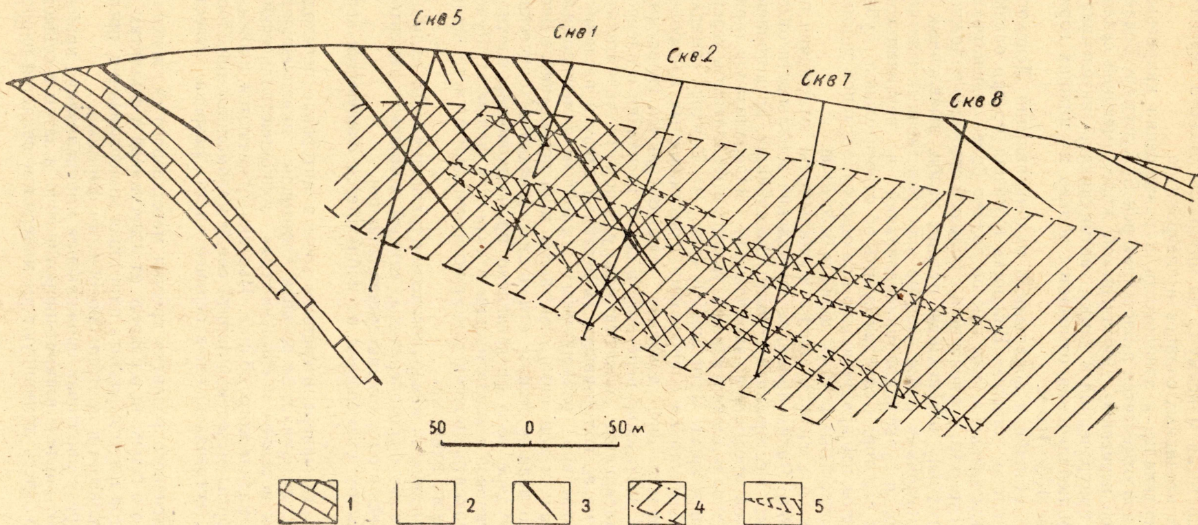
Рис. 3. 1 — переслаивание известковистых алевролитов, известково-глинистых сланцев и известняков; 2 — углистые кварц-серицитовые сланцы (филлиты); 3 — кварцевые жилы; 4 — зона пиритовой прожилково-вкрапленной минерализации; 5 — участки обогащенных золотых руд; 6 — скважины колонкового бурения
