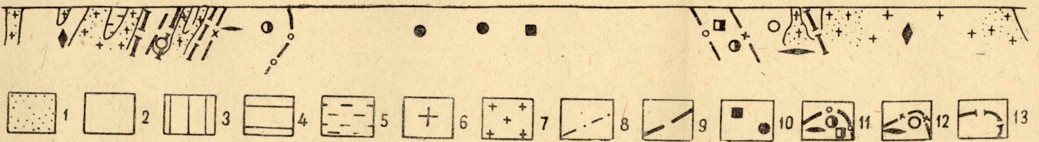
Рис. 1. 1 — илигирская свита, 2 — бодайбинская подсерия, 3 — кадаликанская подсерия, 4 — баллаганахская серия, 5 — мамская серия, 6 — Конкудеро-Мамаканский интрузивный комплекс (Pz), 7 — Мамско-Оронский интрузивный комплекс (Pt 3 ), 8 — тектонические нарушения, 9 — зона глубинного разлома по геолого-геофизическим данным, 10 — зона золотоносных кварцевых жил с полиметаллической минерализацией и золотоносных сульфидных (пиритовых) «минерализованных зон», 11 — зона «пустых» кварцевых жил (вещающие породы слабо минерализованы пирротином), 12 — зона слабозолотоносных кварцевых жил с пирит-пирротиновой минерализацией (вещающие породы несут пирит-пирротиновую минерализацию), 13 — зона слюдоносных пегматитов
