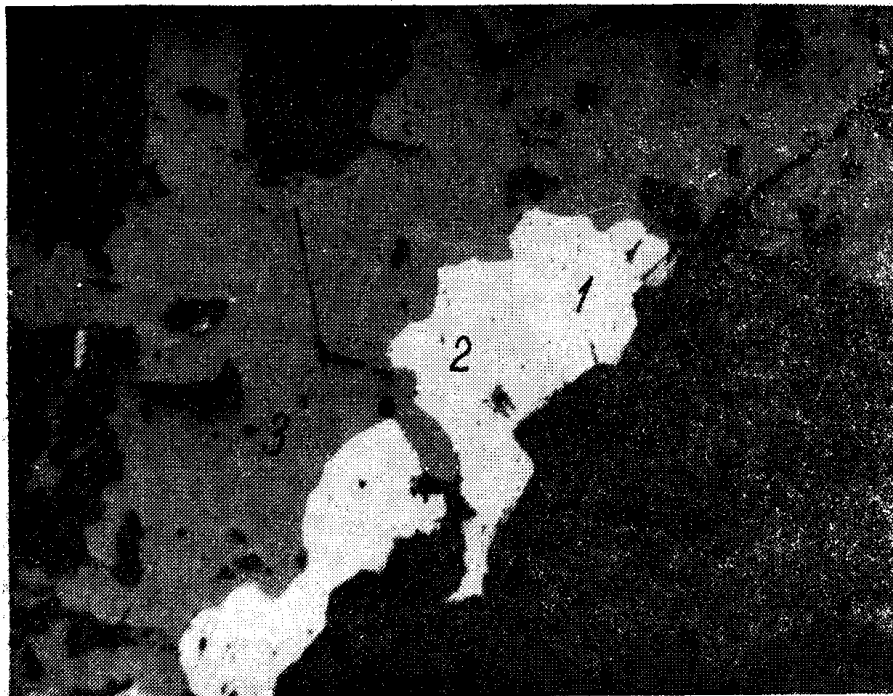
Рис. 3. Срастание золота (1) с галенитом (2) на границе сфалерита (3) с нерудными минералами (черное). Аншлиф 3280/5, увел. 600.
