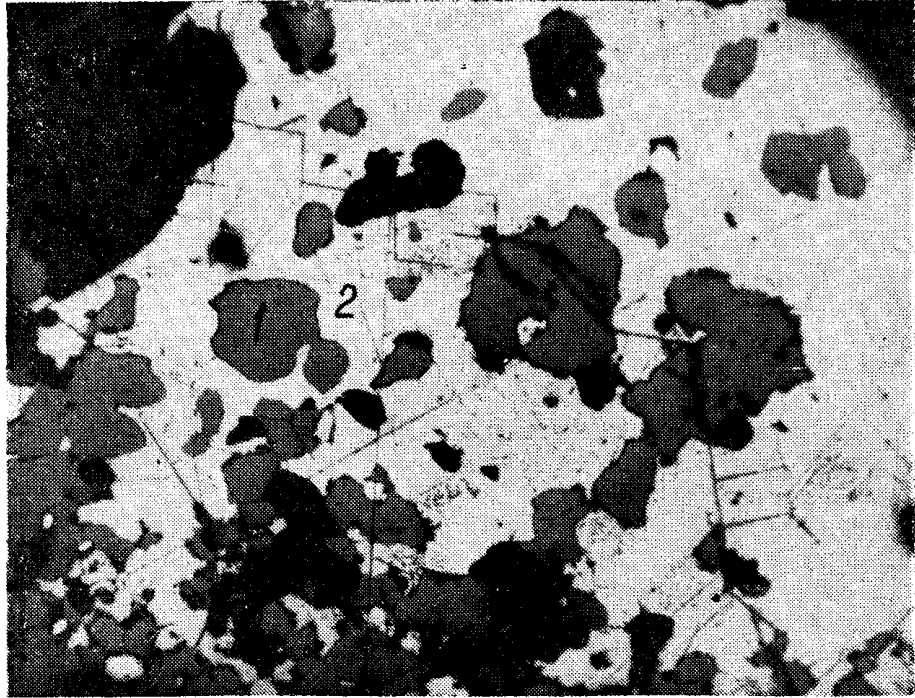
Рис. 1. Замещение сфалерита (1) галенитом (2) в листованите. Аншлиф 3278/6, увел. 250.
