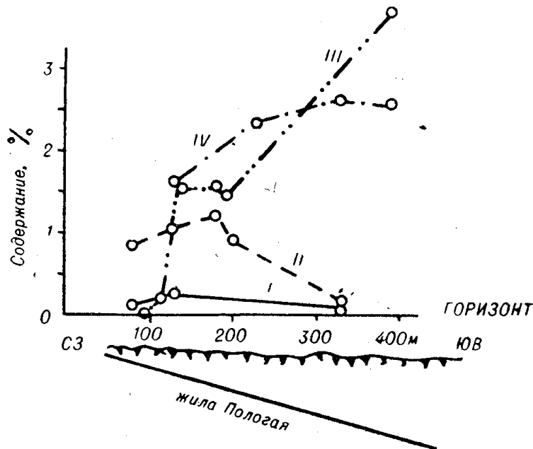
Рис. 1. Пространственное распределение суммарного содержания элементов-примесей в минералах III и IV стадий, I — арсенопирит, II — пирит, III — сфалерит, IV — галенит.
