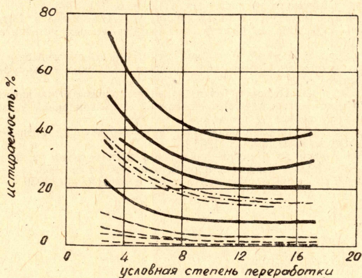
Рис. 2. Зависимость истираемости топливо-плавильных материалов на разных стадиях пиролиза от степени переработки торфа с различной исходной влажностью.
