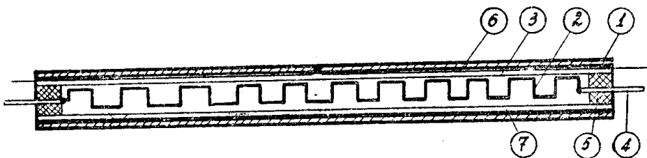
Рис. 2. 1—латунная трубка; 2—нагреватель нихромовый; 3—стеклянная трубка; 4—мелкий токоподвод к нагревателю; 5—жаростойкая замазка; 6—термопара; 7—кольцевое пространство, заполненное алюминиевой фольгой.
