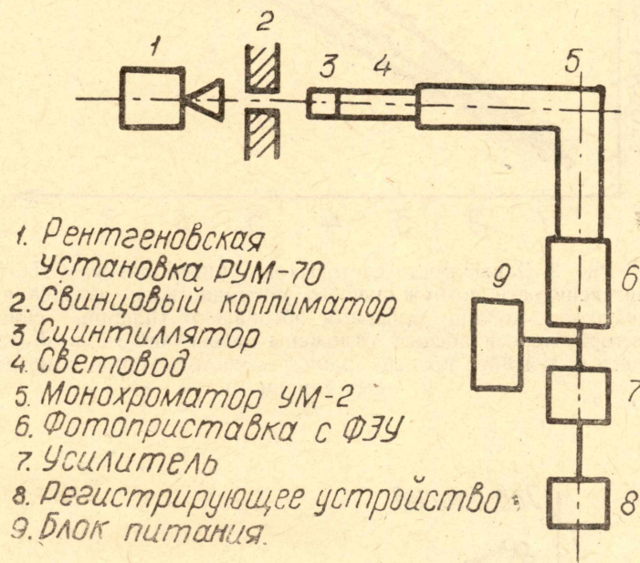
Рис. 1. Блок-схема установки.
