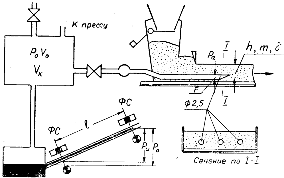
Рис. 2. Схема подачи воздуха через исследуемую пробу.
