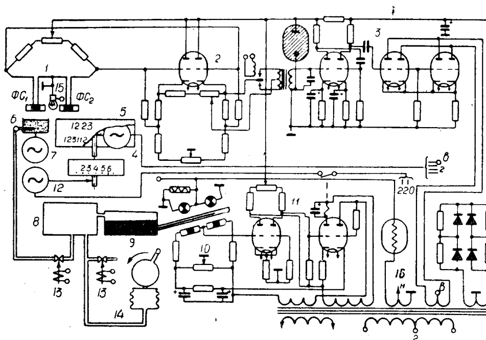
Рис. 1. Принципиальная схема прибора: \Phi C_1 , \Phi C_2 — фотосопротивления; 1 — измерительный мост; 2 — катодный повторитель; 3 — электронный усилитель; 4 — реверсивный двигатель; 5 — диск с набором эталонных проб; 6 — исследуемая проба; 7 — двигатель подачи пробы; 8 — камера; 9 — микрометр; 10 — измерительный мост на \Phi C ; 11 — электронный усилитель; 12 — двигатель со шкалой; 13 — электромагнитные клапаны; 14 — пресс; 16 — блок питания.
