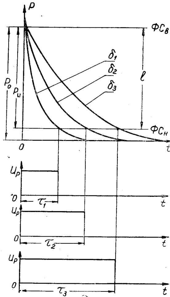
Рис. 3. График зависимости длительности импульса \tau от диаметра частиц \delta .
