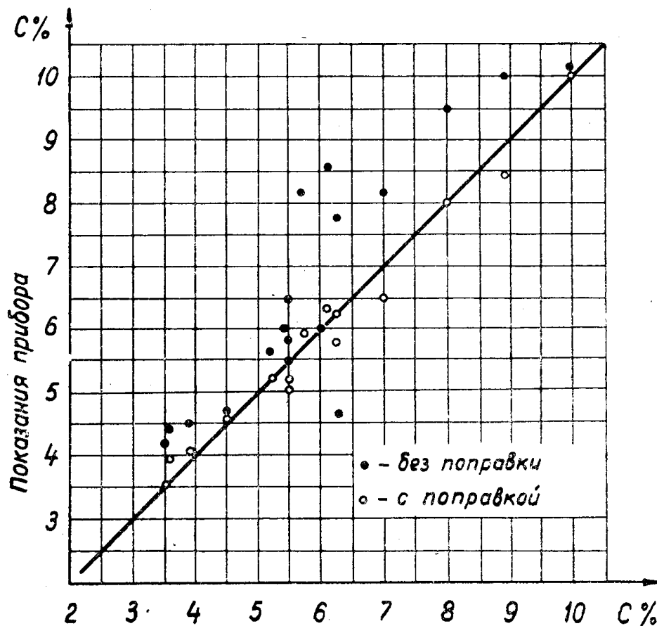
Рис. 5. Показания прибора с поправкой на гранулометрический состав.
