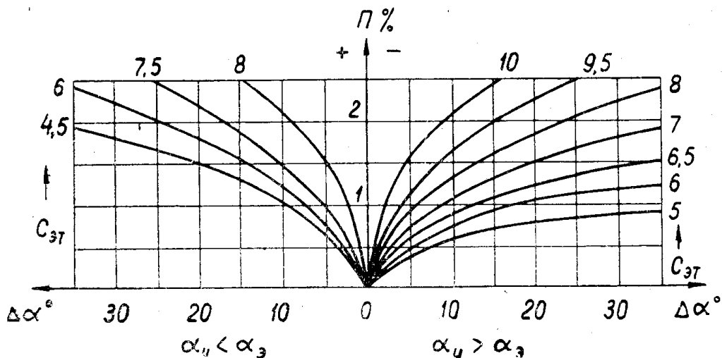
Рис. 4. График для получения поправки П при \alpha_n неравного \alpha_3 .
