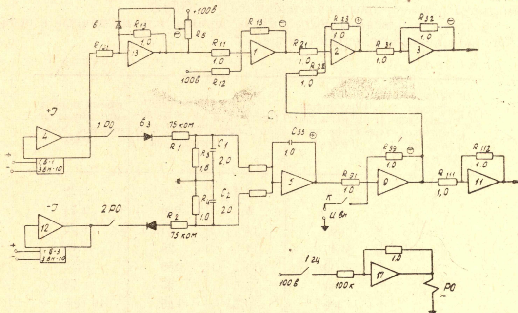
Рис. 2. Электронная модель экстремального регулятора бетатрона. Характеристика бетатрона. При этом масштабы имеют значения: масштаб по интенсивности m_I = 16,6 \frac{\text{отн. ед}}{\text{В}} ; масштаб по фазе (времени) инжекции m_T = 0,17 \frac{\text{мксек}}{\text{В}} . Схема модели регулятора изображена на рис. 2, где обозначение блоков совпадает с обозначением их на модели МН-7.
