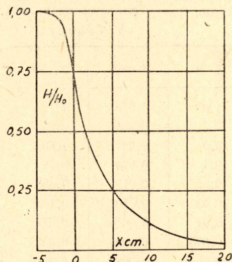
Рис. 4. Кривая спада магнитного поля вдоль расчетной траектории центрального луча при входе в основное магнитное поле.
