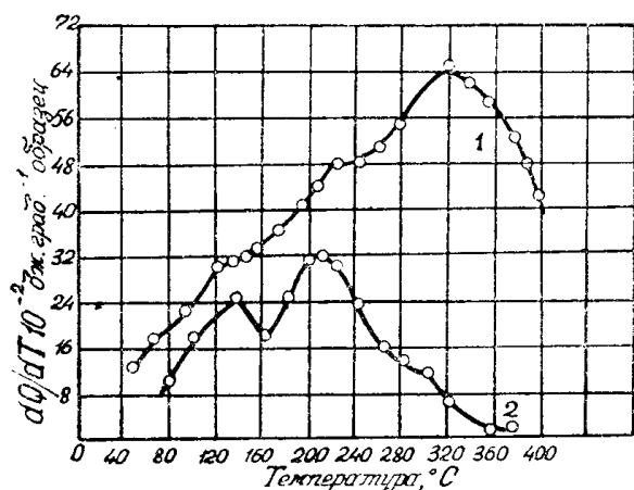
Рис. 1. Спектры выделения запасенной энергии в кристаллах \text{CaF}_2 после облучения рентгеновскими (кривая 2) и гамма-лучами (кривая 1) при нагревании до 400°C.
