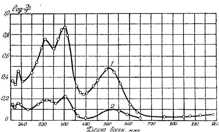
Рис. 2. Спектры поглощения кристаллов \text{CaF}_2 после облучения рентгеновскими (кривая 2) и гамма-лучами (кривая 1).
