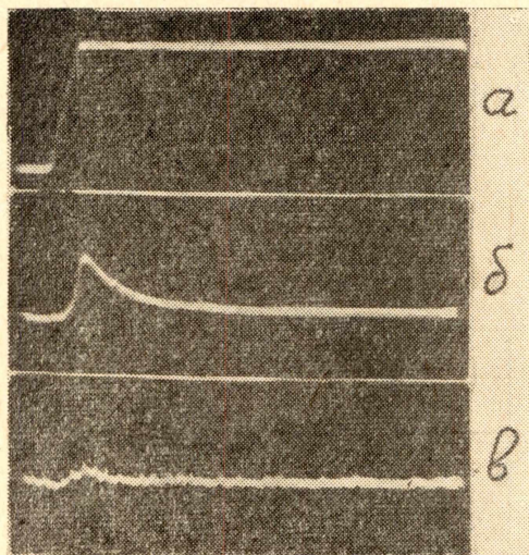
Рис. 2. Осциллограммы напряжения и токов; a — приложенное импульсное напряжение; b — ток в первом импульсе; v — ток во втором импульсе (токи измерялись в образце твердого раствора 10 мол % КВг в КС1).
