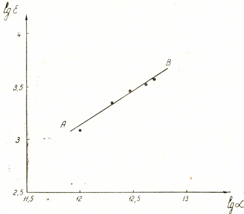
Рис. 1. К аппроксимации зависимости мощности эхо-сигнала \Sigma от линейной плотности электронов \alpha в ионизированном следе (для радиоэхо промежуточного типа). Точки — теоретический результат [3]; AB — аппроксимирующая линия.
