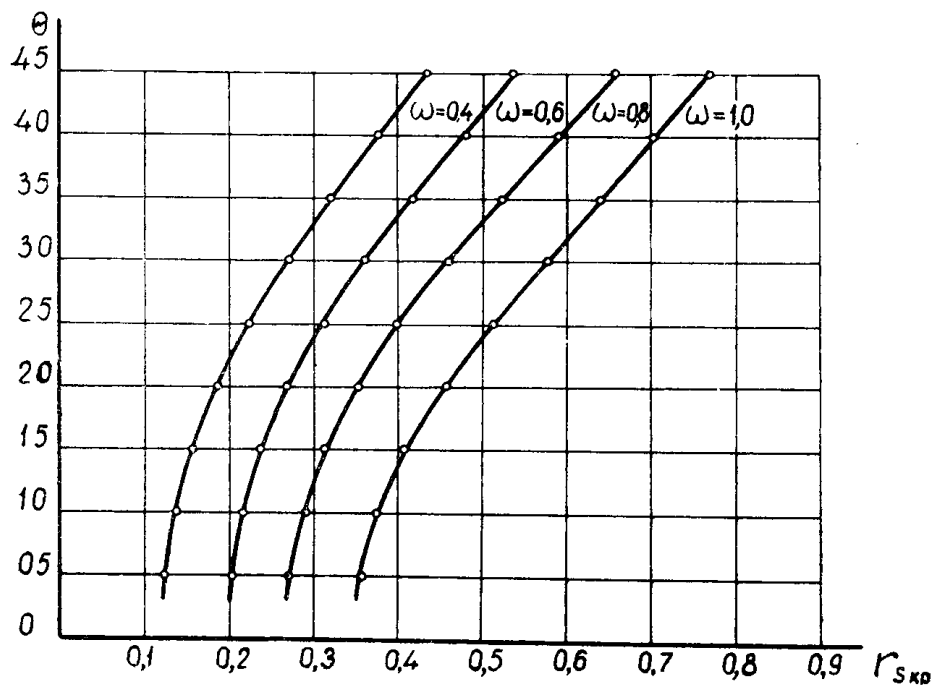
Рис. 3. Влияние нагрузки синхронно-реактивного двигателя на расположение границы области устойчивой работы.
