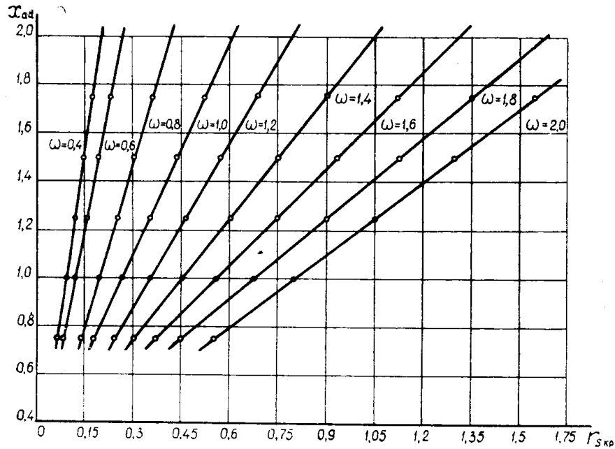
Рис. 1. Влияние сопротивления x_{ad} на расположение границы области устойчивой работы при \frac{x_{ad}}{x_{aq}} = \text{const} .
