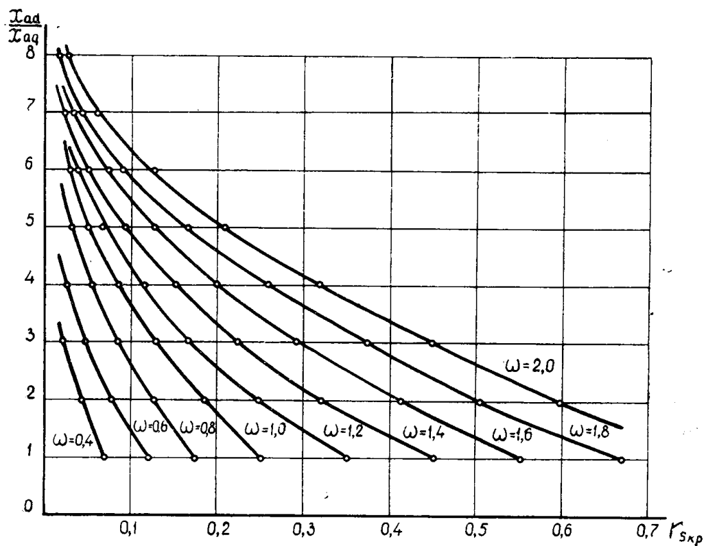
Рис. 2. Влияние отношения \frac{x_{ad}}{x_{aq}} на расположение границы области устойчивой работы при x_{ad} = \text{const} .
