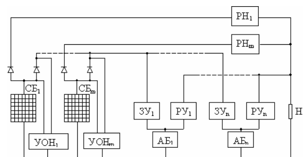
Рис. 1 Система электроснабжения с секционированной СБ
