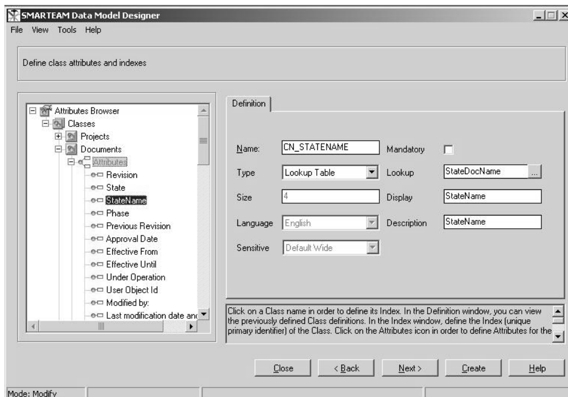
Рис. 4 Этап проектирования МД, окно определения атрибута «Состояние ЖЦ»
