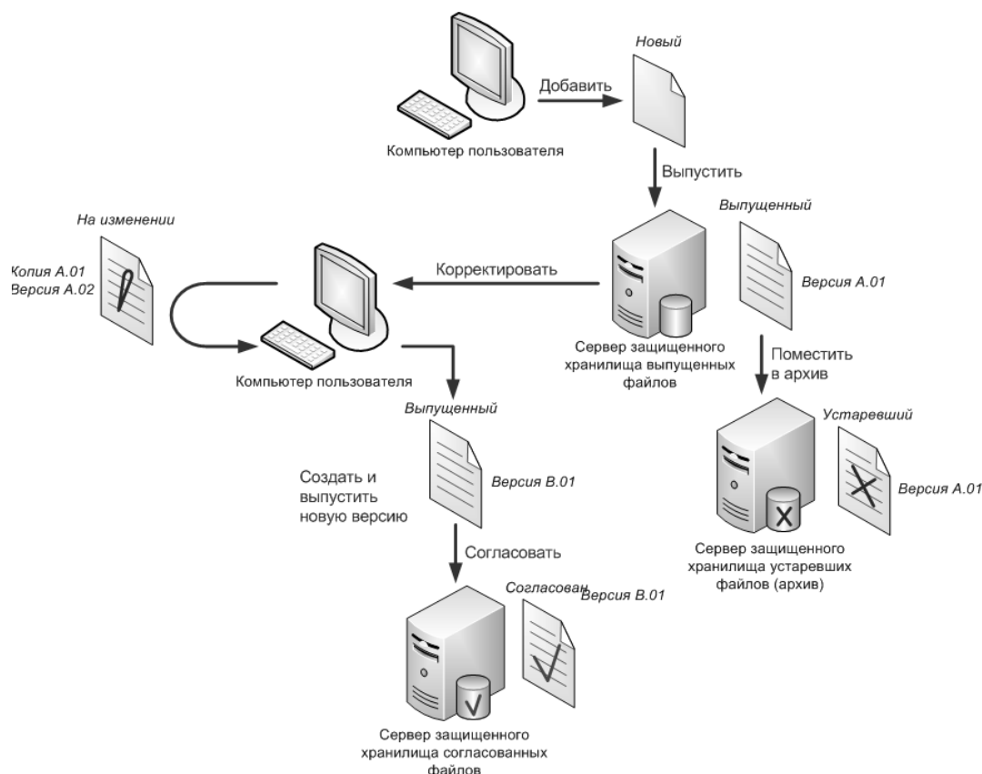
Рис. 2. ЖЦ документа в PDM-системе Enovia SmartTeam
