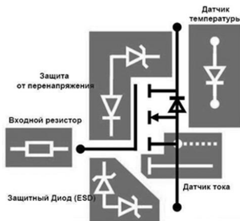
Рис. 1. Схема функционального устройства современных MOSFET
