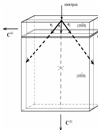
Рис. 1. Схема возбуждения разрядов и взаимная ориентация защитного (буферного) (а) и рабочего (б) кристаллов CdS в импульсно-периодическом режиме
