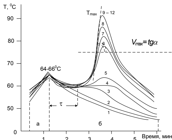
Рис. 1. Изменение температуры во времени при взаимодействии нанопорошка алюминия с водой: а) одновременное нагревание и перемешивание суспензии; б) только перемешивание суспензии; \tau – индукционный период, мин; V_{\max} – максимальная скорость роста температуры, °С/с; T_{\max} – максимальное значение температуры суспензии (воды); 1, 2, ..., 12 – номера суспензий с различным содержанием нанопорошка алюминия (табл.)
