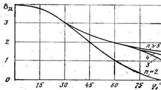
Рис. 3. Допустимый показатель колебательности
