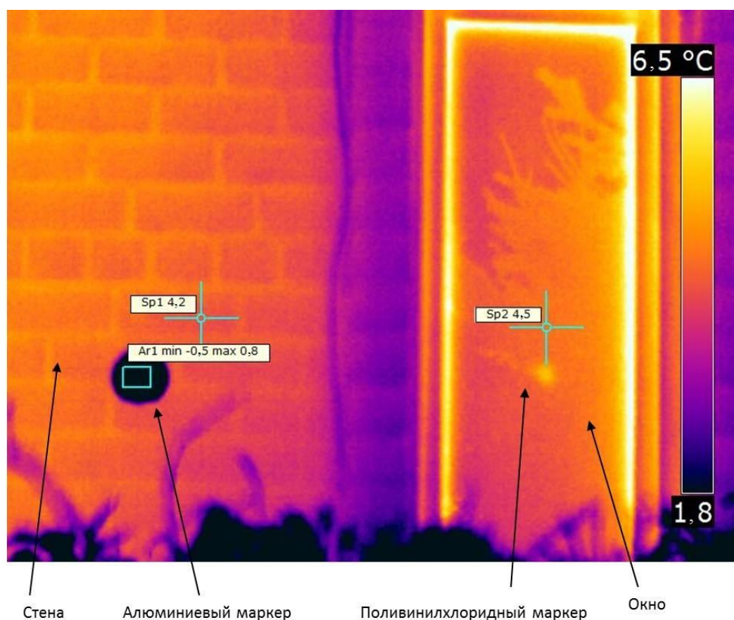
Рисунок. ИК термограмма, иллюстрирующая экспериментальную процедуру
