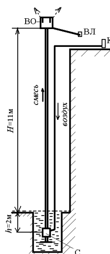
Рис. 2. ВО – вододетектор, ВЛ – водяной лоток, К – компрессор с избыточным давлением 0,3 ати, производительностью 5 м 3 /мин, С – смеситель.
