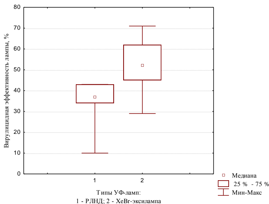
Рис. 3. Эффективность инактивации фага MS2 УФ-излучением РЛНД и ХеВг-эксиллампы
