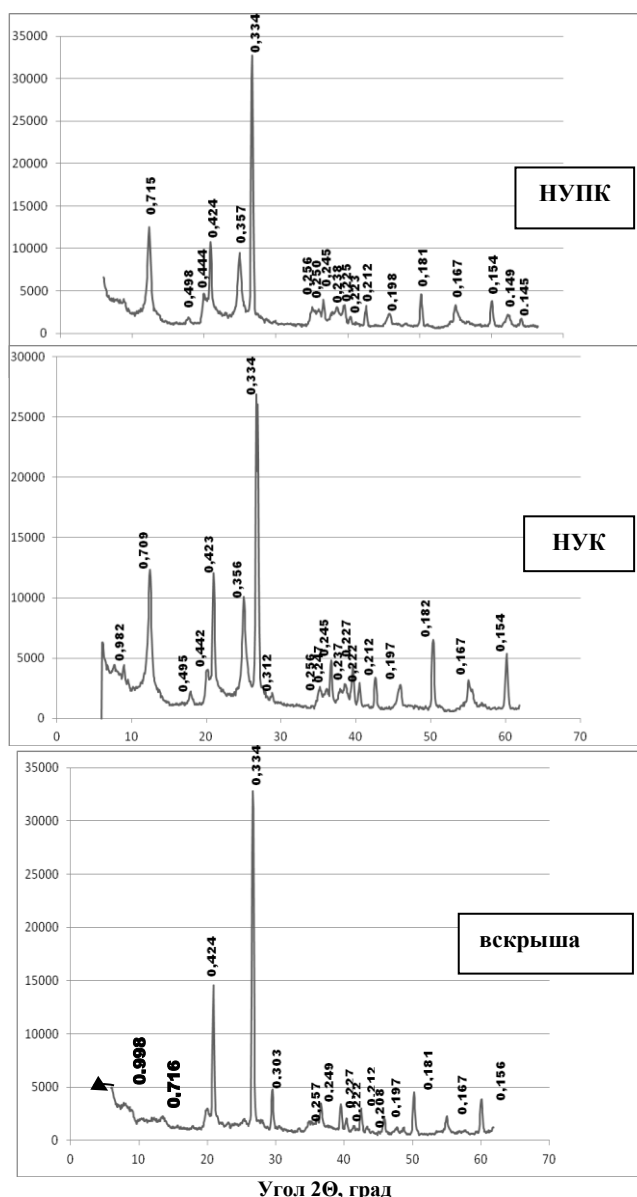
Рис. 1. Рентгеновские дифрактограммы нижеуевельских глин
