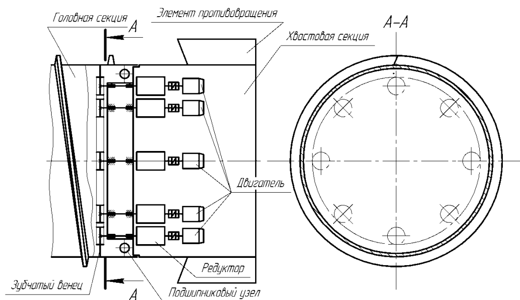
Рис. 4. Кинематическая схема трансмиссии геохода с многопоточным редукторным приводом
