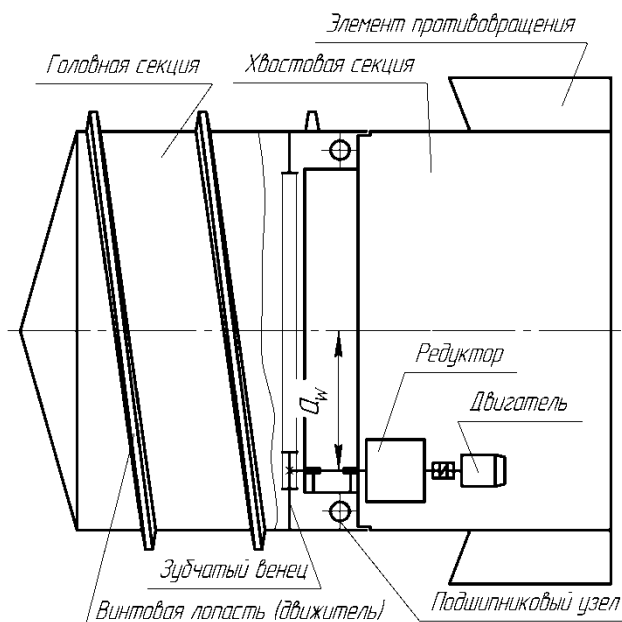
Рис. 1. Кинематическая схема трансмиссии геохода с редукторным приводом
