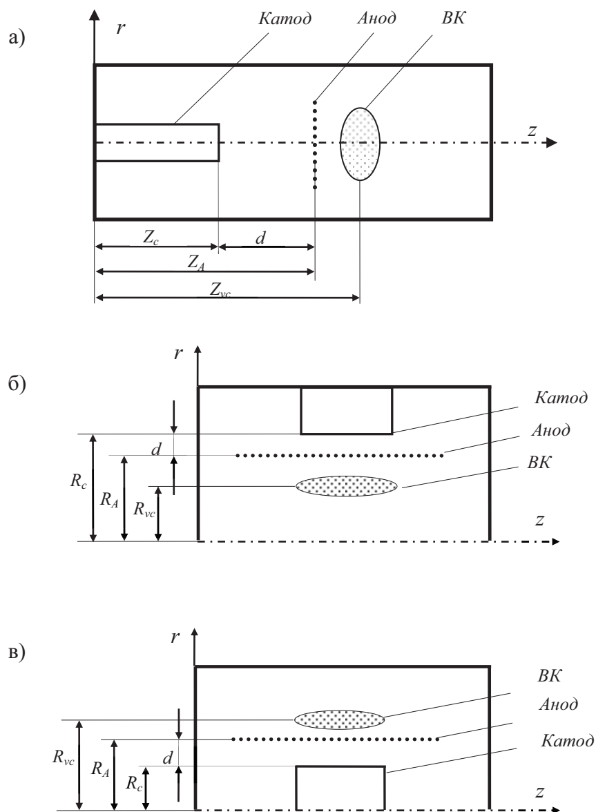
Рис. 1. Схемы отражательных триодов: а) триод с планарной конфигурацией электродов; б) коаксиальный триод с радиально-сходящимся пучком; в) коаксиальный триод с радиально-расходящимся пучком
