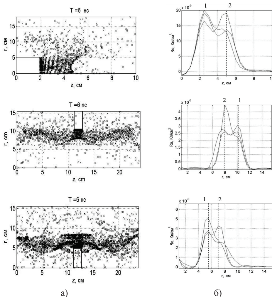
Рис. 2. Конфигурационные портреты пучка (а) и распределение плотности заряда вдоль координаты движения пучка в триодных системах (б); U_0 = 450 кВ
