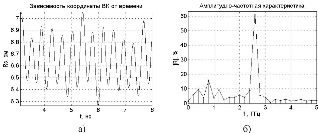
Рис. 3. Зависимость усредненной координаты виртуального катода от времени (а) и амплитудно-частотная характеристика колебаний ВК (б) коаксиального триода; U_0 = 450 кВ
