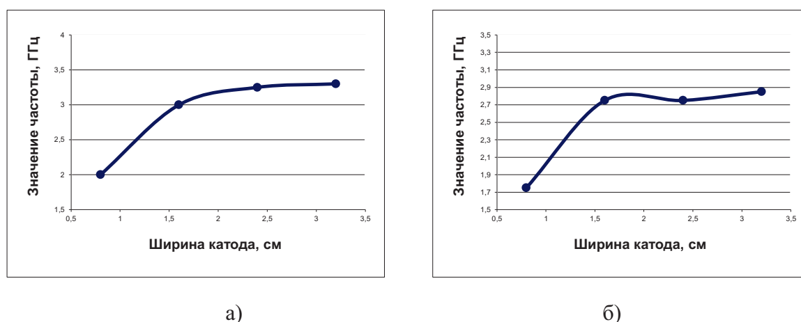
Рис. 5. Зависимость частоты колебаний ВК в коаксиальном триоде: а) сходящийся пучок; б) расходящийся пучок
