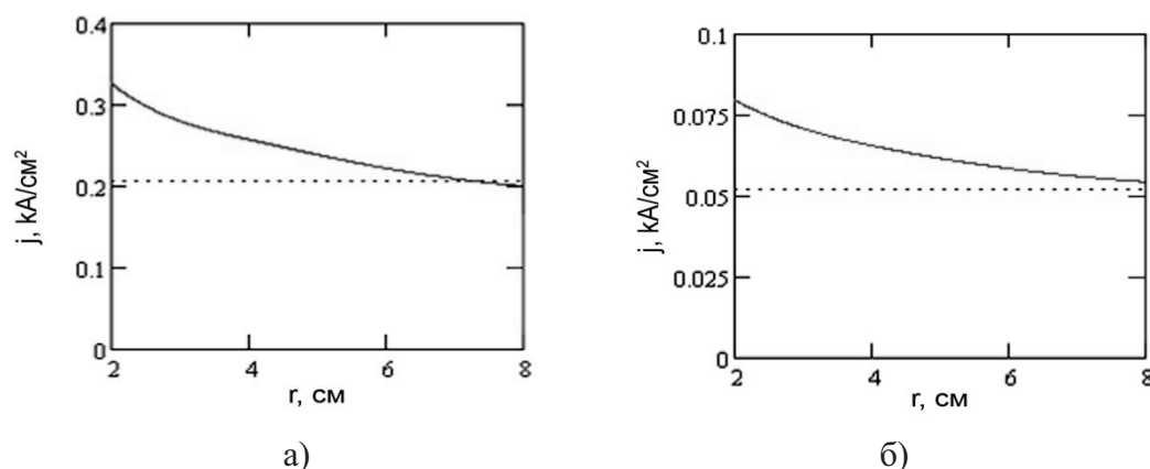
Рис. 4. Зависимость плотности тока от радиуса пучка в планарном (—) и одномерном (··) триодах: а) U_0 = 200 кВ; б) U_0 = 500 кВ
