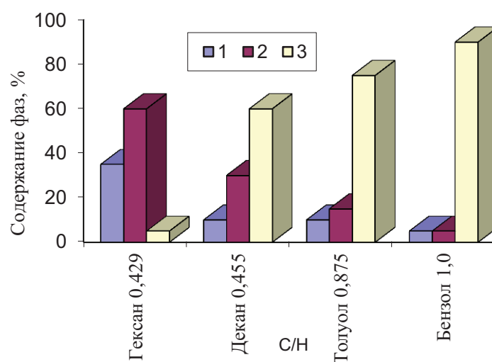
Рис. 4. Содержание фаз W (1), W_2C (2), и WC_{1-x} (3) в продуктах электрического взрыва вольфрамовых проводников в зависимости от соотношения С/Н в молекулах углеводородов
