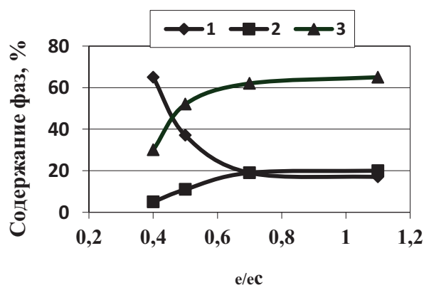
Рис. 5. Зависимость относительного содержания W (1), W_2C (2) и WC_{1-x} (3) в продуктах электрического взрыва вольфрамовых проводников в декане от введенной в проводник энергии
