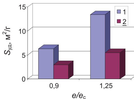
Рис. 6. Влияние удельной введенной в проводник энергии на площадь удельной поверхности порошков карбида тантала, полученных в ацетилен-аргоновых смесях с молярным соотношением 4:1 (1) и 9:1 (2)
