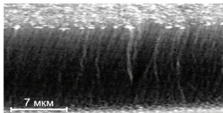
Рис. 3. РЭМ-изображение скола слоя высокоориентированных углеродных нанотрубок, сформированных на кремниевой подложке путем осаждения из газовой фазы
