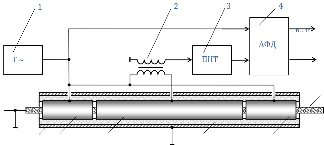
Рис. 1. Структурная схема измерителя емкости: 1 – генератор; 2 – трансформатор тока; 3 – преобразователь ток–напряжение; 4 – амплитудно-фазовый детектор; 5 – корпус преобразователя; 6 – измерительный электрод; 7 – дополнительные электроды; 8 – диэлектрик; 9 – кабель
