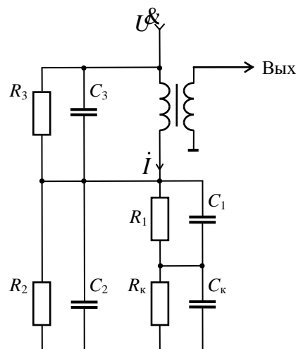
Рис. 2. Схема замещения электрической цепи измерительного электрода: C_1 и R_1 – емкость и активное сопротивление между измерительным электродом и диэлектрической оболочкой кабеля; C_2 и R_2 – емкость и активное сопротивление между измерительным электродом и землей (корпусом преобразователя и стенками охлаждающей ванны); C_3 и R_3 – емкость и активное сопротивление между измерительным и дополнительными электродами
