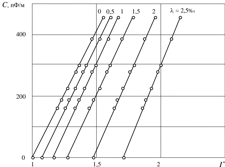
Рис. 4. Зависимость относительного амплитудного значения тока I^* от погонной емкости кабеля C и солёности воды \lambda
