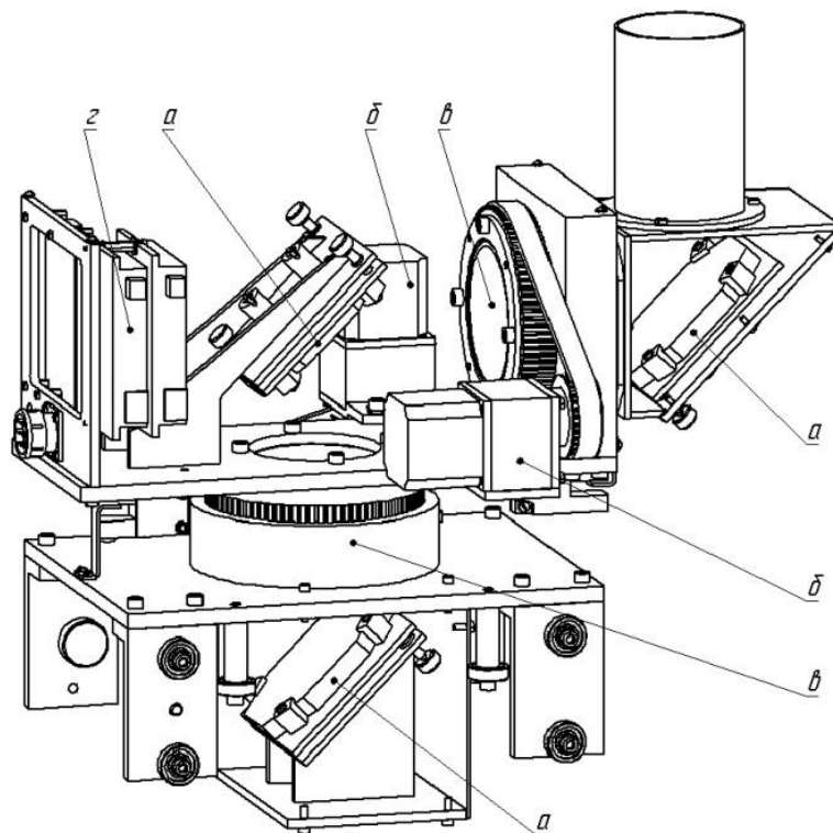
Рис. 2. Схематический вид трекера: а) зеркала; б) шаговые двигатели; в) полые оси вращения; г) стойка с электроаппаратурой
