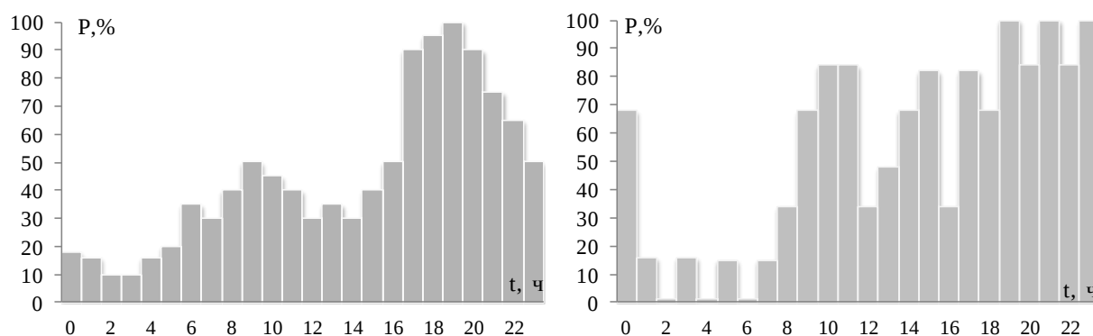
Рис. 3. Суточный график коммунально-бытовой нагрузки и ЗЖБИ
