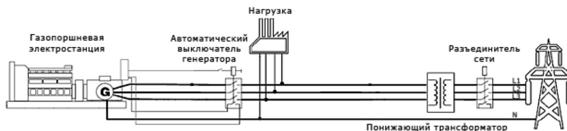
Рис. 2. Подключение ГПУ через трансформатор [6]
