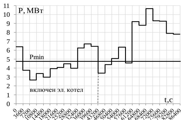
Рис. 6. Суточный график нагрузки при подключенном котле
