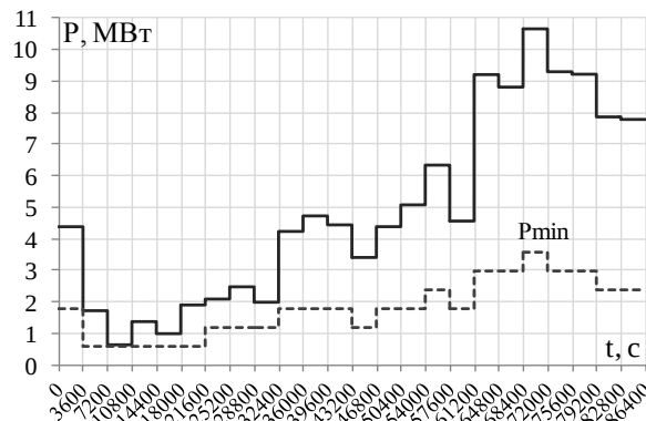
Рис. 7. График нагрузки при ОГ
