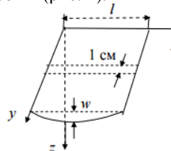
Рисунок 2 - Мембрана прямоугольной формы
