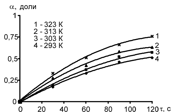
Рис. 5. Кинетика взаимодействия 3 % раствора \text{NH}_4\text{OH} и (\text{NH}_4)_2\text{SiF}_6
