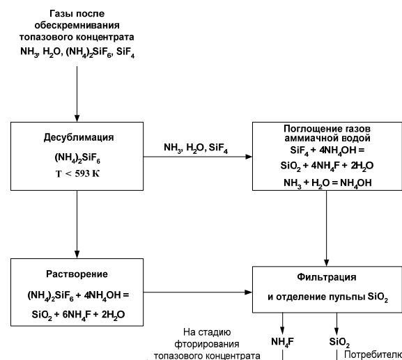
Рис. 2. Принципиальная схема утилизации фторсодержащих газов
