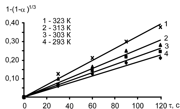
Рис. 6. Обработка кинетических кривых по уравнению сокращающейся сферы
