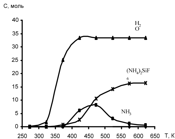
Рис. 1. Равновесный состав газовой фазы
