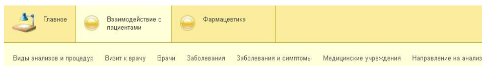
Рис. 1. Основные разделы
