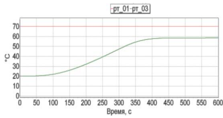
Рис. 1. Критическая продолжительность пожара по повышенной температуре
