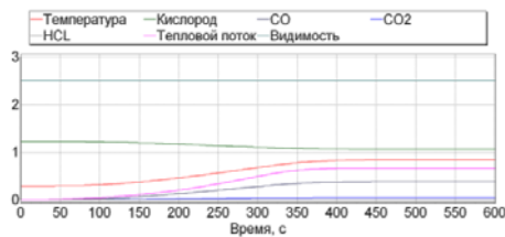
Рис. 10. Развитие всех опасных факторов пожаров
