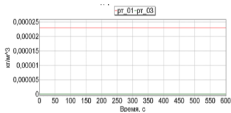
Рис. 6. Критическая продолжительность пожара по содержанию соляной кислоты
