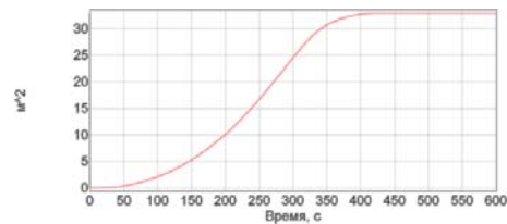
Рис. 11. Площадь развития пожара
