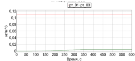
Рис. 4. Критическая продолжительность пожара по содержанию углекислого газа
