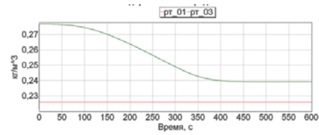
Рис. 2. Критическая продолжительность пожара по содержанию кислорода
