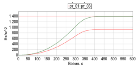
Рис. 7. Критическая продолжительность пожара по тепловому потоку
