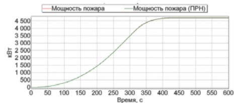
Рис. 9. Развитие мощности пожара
