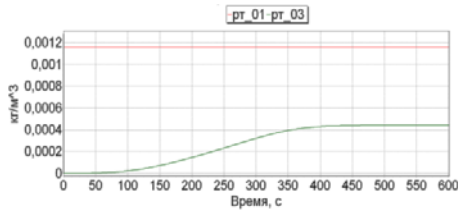
Рис. 3. Критическая продолжительность пожара по содержанию угарного газа
