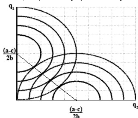
Рис. 2. Изопрофитные кривые
