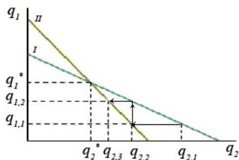
Рис. 1. Равновесие Курно
