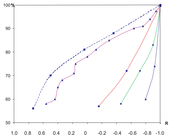
Рис. 2. Радиальное от начала координат движение точек проб при уменьшении содержания в них суммы «фоновых» компонентов. Квадратики – «начальное» положение точек, характеризующее корреляционным эллипсом 1 ( r=0,7 ); кружки – положение точек при уменьшении содержания фоновых компонентов в среднем с 45 до 25 %, корреляционный эллипс превратился в круг 2 ( r=0,0 )
