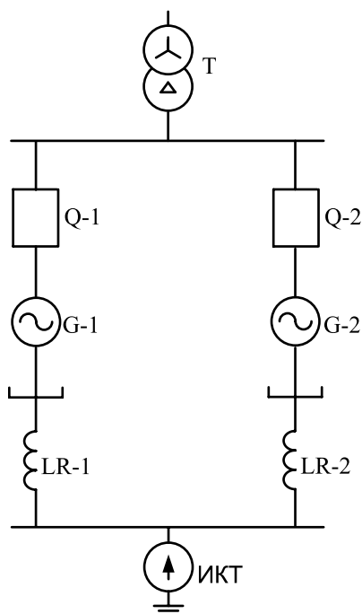
Рис. 1. Схема энергоблока с параллельно включенными генераторами G-1 и G-2
