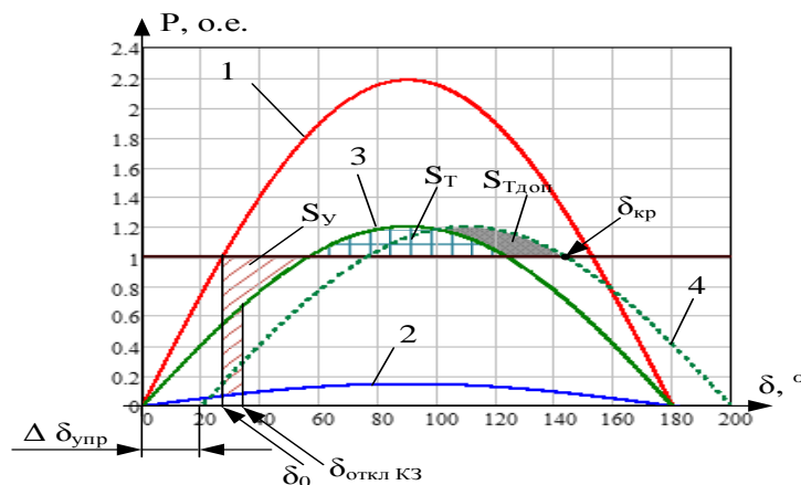
Рис. 2. Угловые характеристики мощности электропередачи
