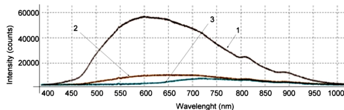
Рис. 3. Спектры прошедшего излучения через объекты. 1 – источника излучения без объекта, 2 – после прохождения через фторопласт, 3 – после прохождения через кость.
