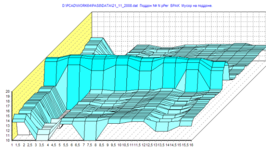
Рис. 2. Результат реконструкции псевдообъемного изображения поверхности паллеты
