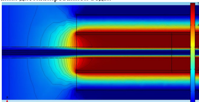
Рис. 3. Картина поля для ЭИИП без дополнительных электродов (вода дистиллированная)
