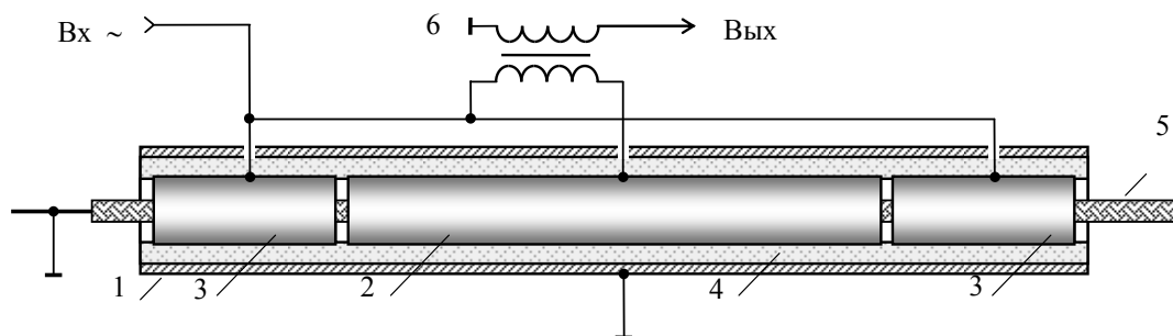
Рис. 1. Конструкция электроемкостного измерительного преобразователя
