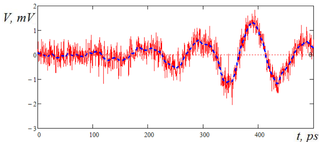
Рис. 5. Разность сигналов
