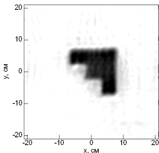
Рис. 5. Восстановленное изображение тестового объекта
