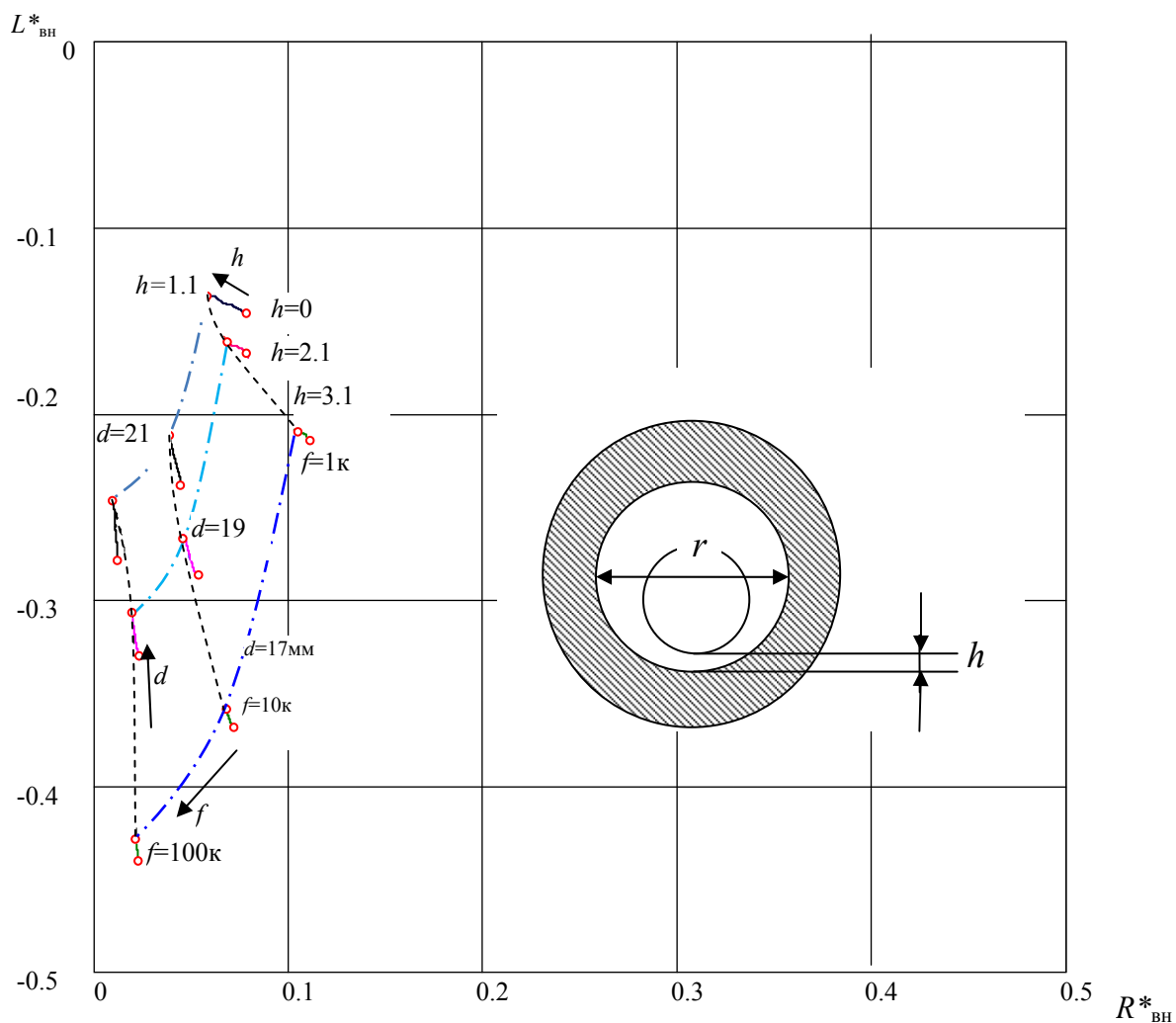
Рис.8. Годографы вносимого сопротивления проходного вихревого преобразователя в трубе от изменения частоты, зазора, внутреннего диаметра трубы
