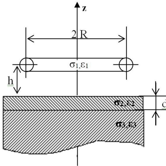
Рис.1. Расчетная модель
