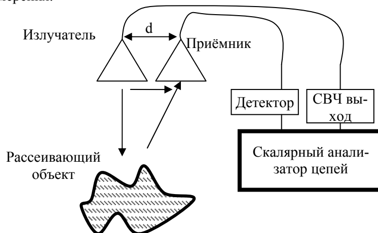
Рис. 1. Схема измерений
