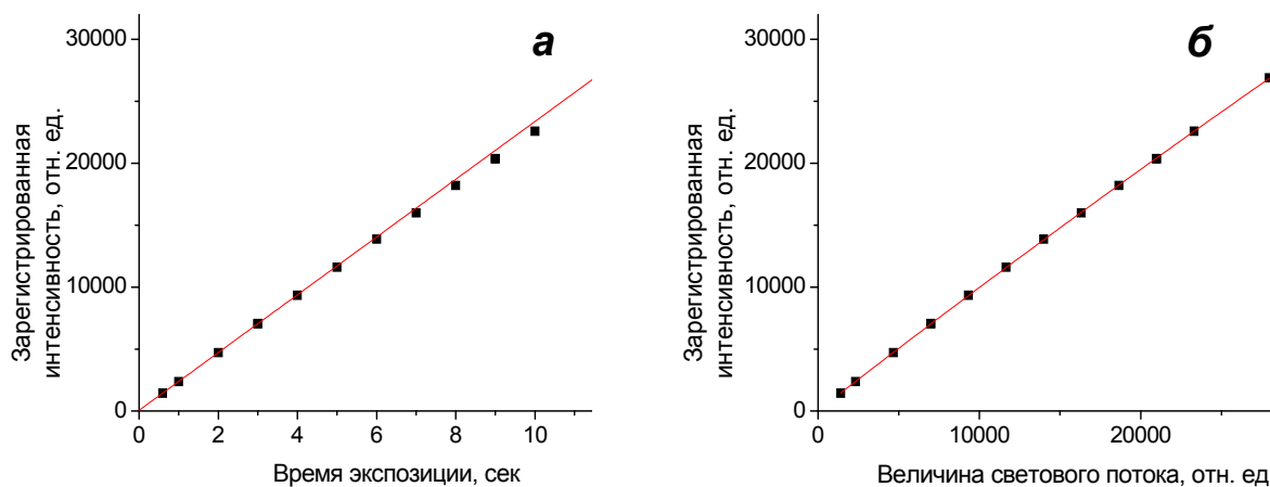
Рис. 4. Зависимость зарегистрированной интенсивности от времени экспозиции одного кадра (а) и от величины светового потока (б)
