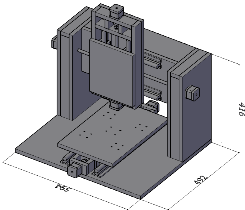
Рис. 5. Габаритный чертеж ЧПУ станка
