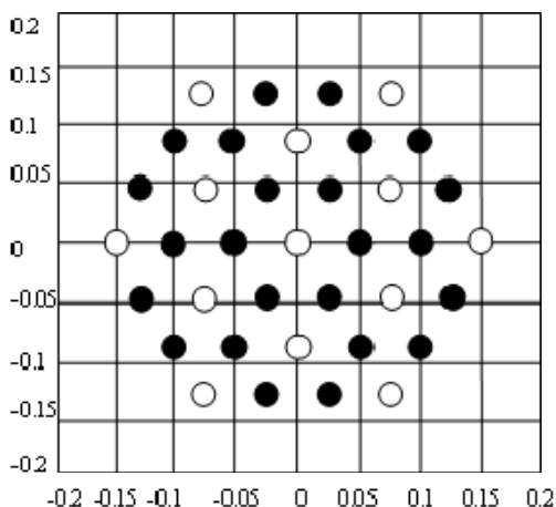
Рис.1. Расположение антенн
