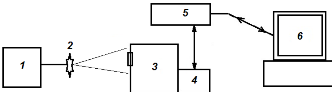
Рис. 2. Блок-схема экспериментальной установки: 1 – блок питания, 2 – лампа накаливания, 3 – спектральный прибор, 4 – ПЗС матрица, 5 – блок управления, 6 – ПК.
