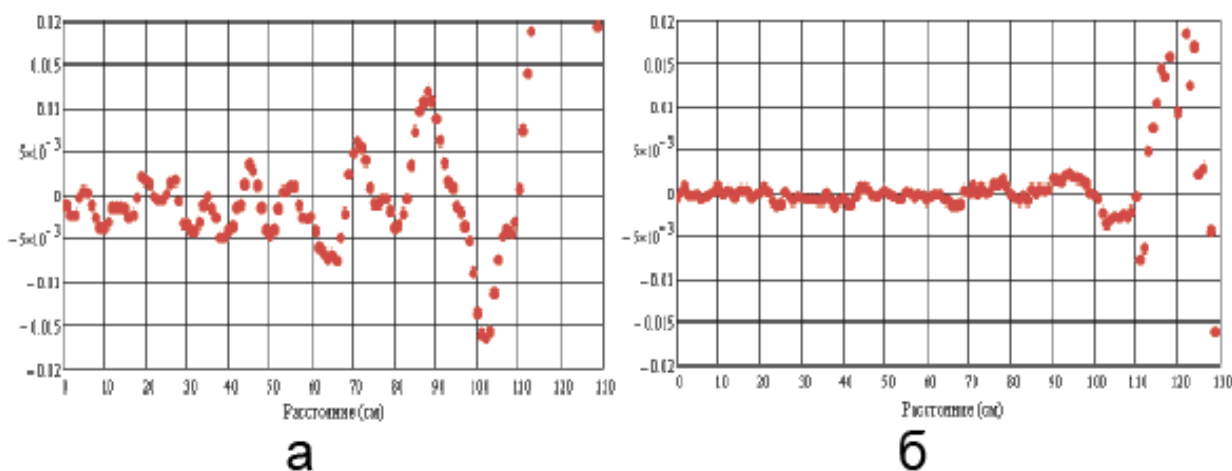
Рис. 7. Оценка погрешности: метода согласованной фильтрации (а), метод линейаризации ФЧХ (б)
