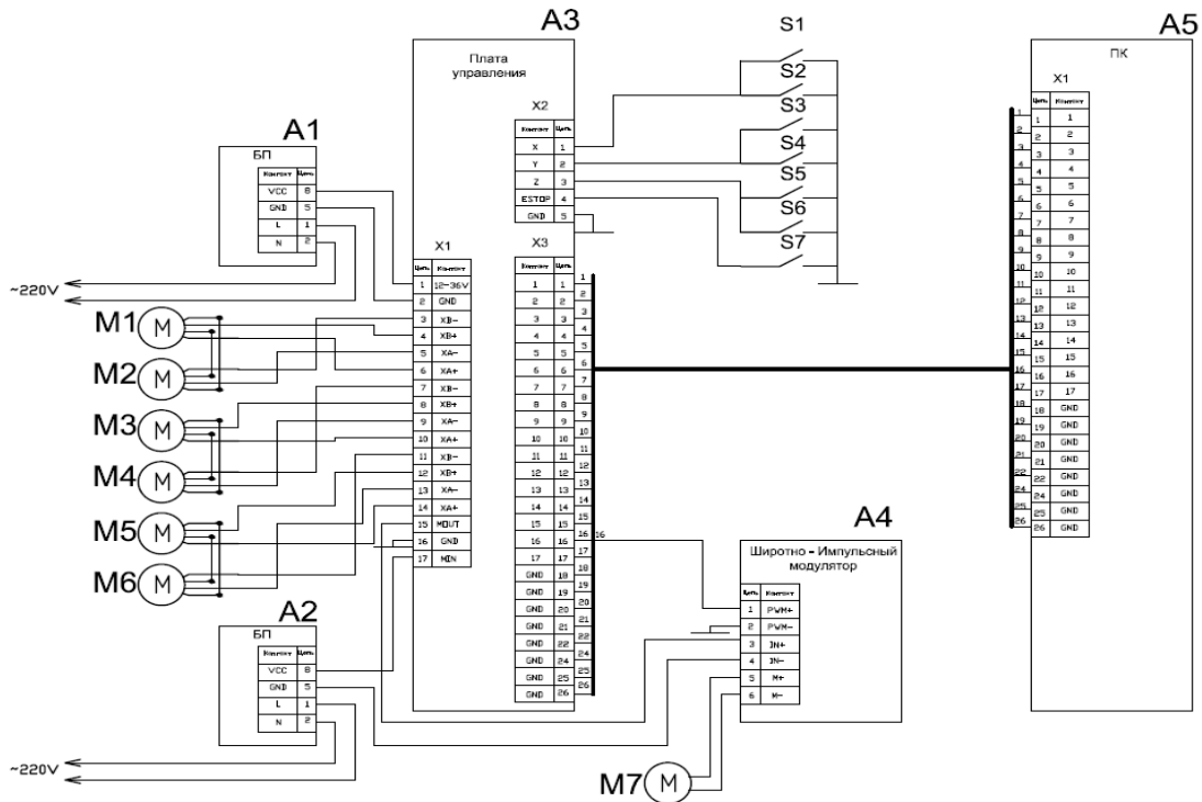
Рис. 1. Принципиальная схема ЧПУ станка
