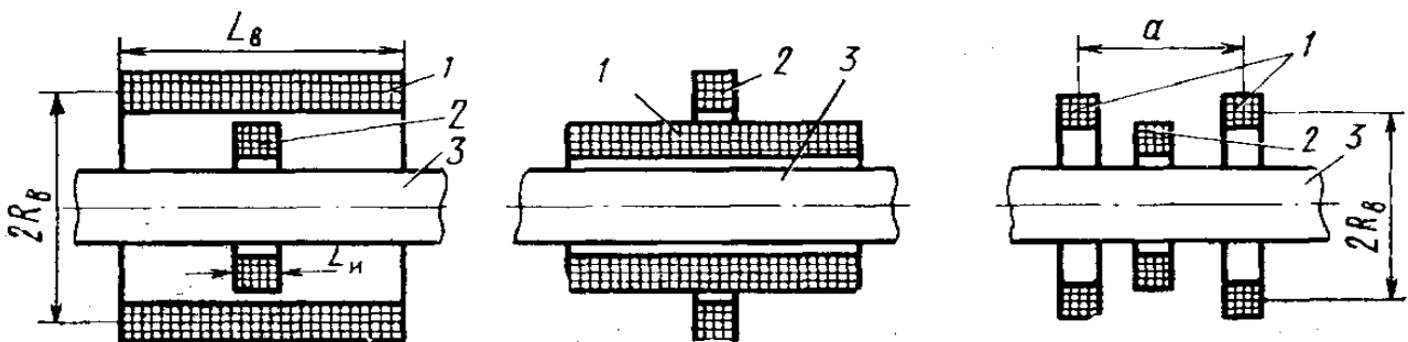
Рис. 3. Проходные наружные ВТП Пер. лист 1
