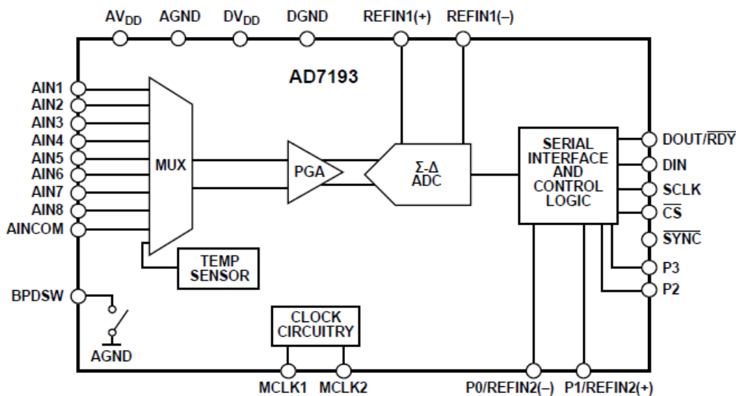
Рис. 2. Функциональная диаграмма AD7193
