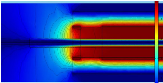
Рис. 8. Картина поля на краю измерительного преобразователя для ЭИИП с дополнительными электродами длиной 0,5R и зазоре 15 мм (вода дистиллированная)
