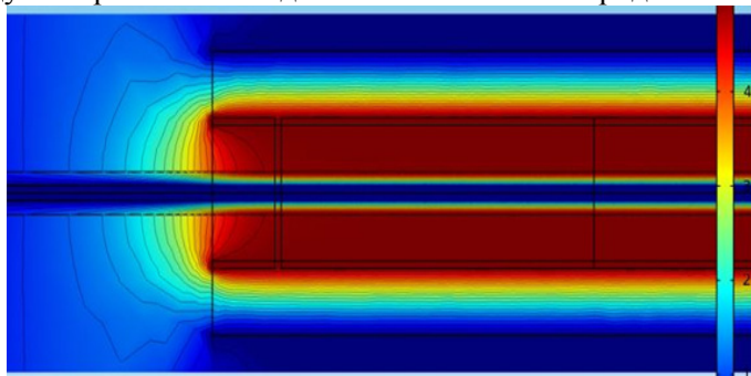
Рис. 5. Картина поля на краю измерительного преобразователя для ЭИП с дополнительными электродами длиной 1R и зазоре 1 мм (вода дистиллированная)
