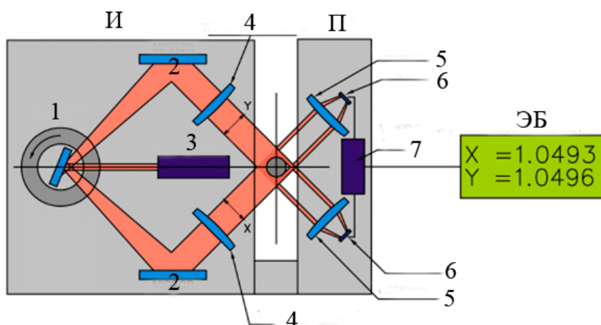
Рис. 1. Принцип сканирования диаметра проводника лазерным прибором: И – излучатель, П – приемник, ЭБ – электронный блок, 1 – вращающееся зеркало, 2 – зеркало, 3 – лазерный диод, 4 – передающая линза, 5 – принимающая линза, 6 – фотодиод, 7 – преобразователь
