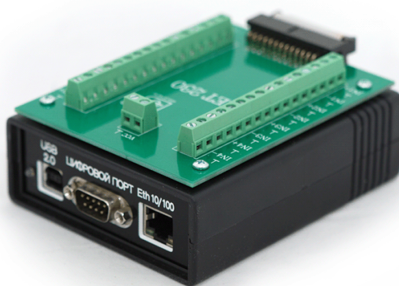
Рис.1. Плата АЦП/ЦАП ZET 230
