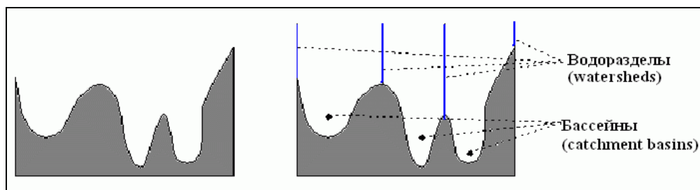
Рисунок 14 – Общая схема понятий алгоритма водораздела
