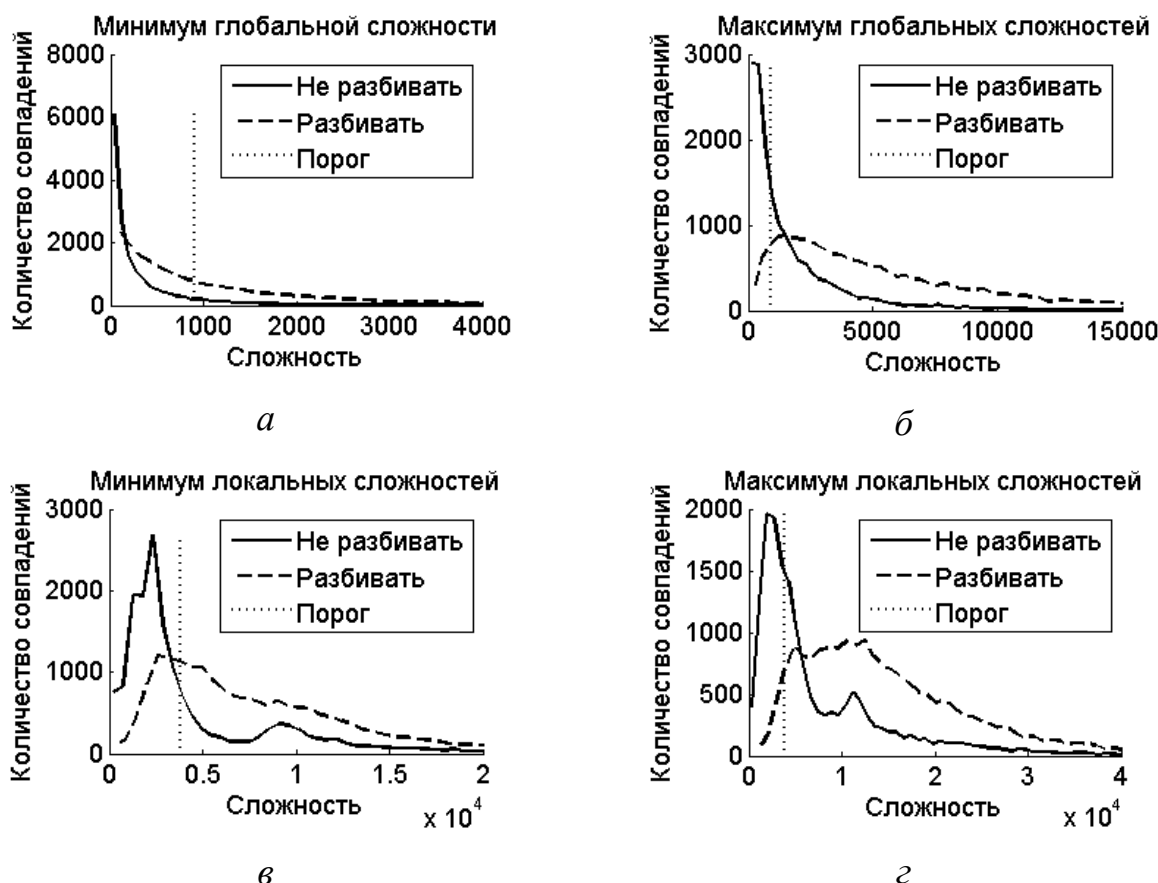
Рисунок 6 – Зависимости количества принимаемых решений от сложности границ ( Q_p = 37 , размер блока – 32 \times 32 ): а – от минимума глобальных сложностей, б – от максимума глобальных сложностей, в – от минимума локальных сложностей, г – от максимума локальных сложностей
