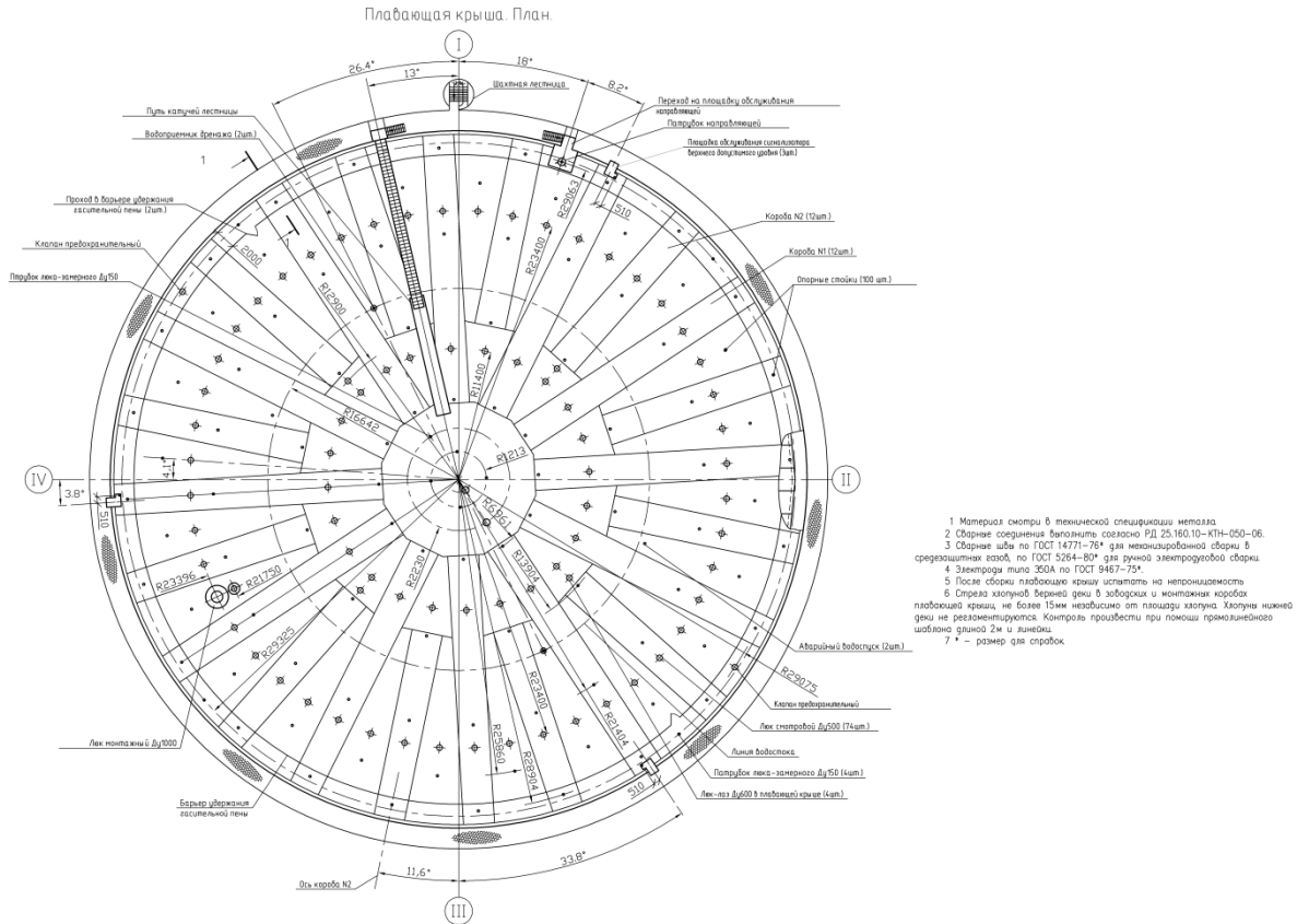
Рисунок Б1 – Схема плавающей крыши
