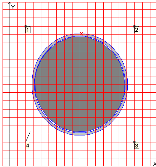
Рисунок 5.8 – Схема площадки
